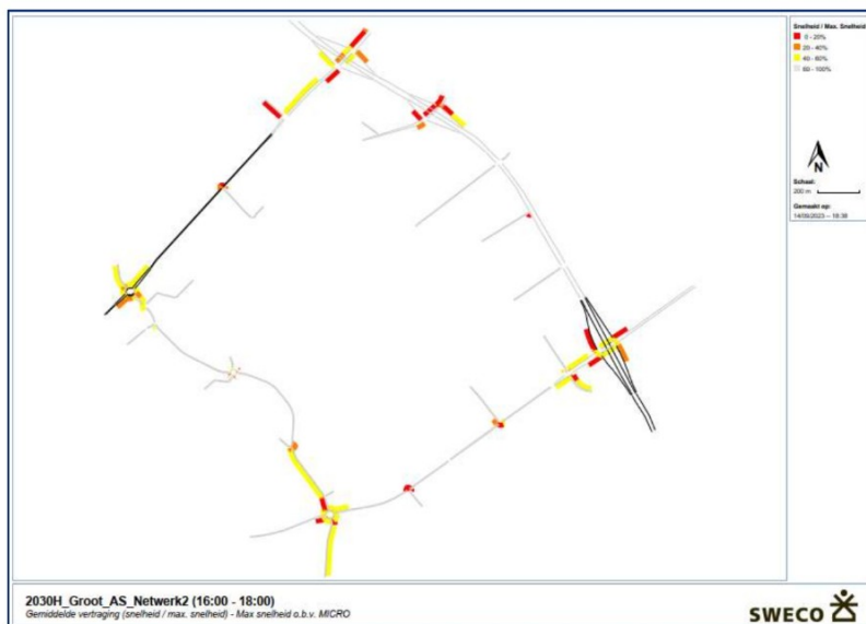
Fig. 15. Verkeersafwikkeling in de avondspits 2040 met geoptimaliseerde kruisingen, inclusief uitbreiding ABC Westland
